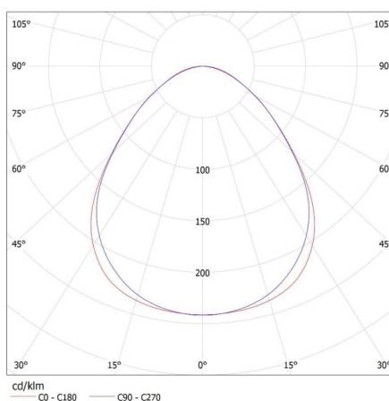
KANLUX S.A. (kat 28451) AL 4LED 120-MPR-SR + Miledo / LDC (Polar)
