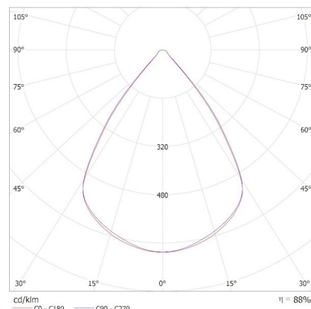
KANLUX S.A. (kat 33908) AL-SL-NW-RST-W-NT / Krzywa rozsyłu światła (biegunowo)
