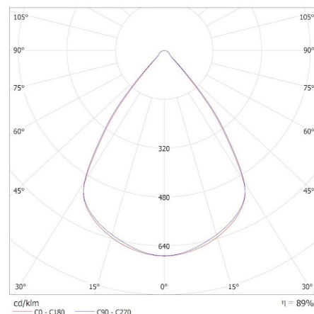
KANLUX S.A. (kat 33909) AL-SH-NW-RST-W-NT / Krzywa rozsyłu światła (biegunowo)
