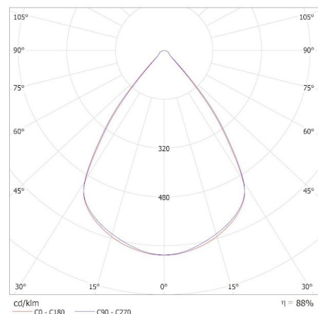
KANLUX S.A. (kat 33910) AL-SL-WW-RST-W-NT / Krzywa rozsyłu światła (biegunowo)
