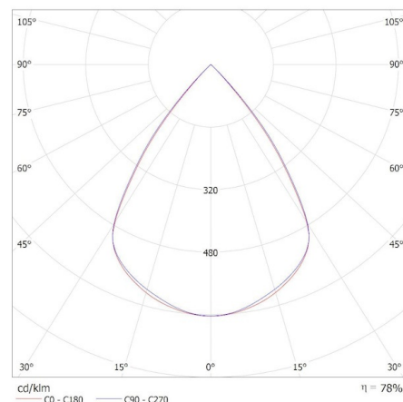
KANLUX S.A. (kat 33920) AL-SL-NW-RST-B-NT / Krzywa rozsyłu światła (biegunowo)
