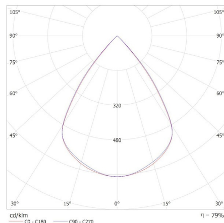
KANLUX S.A. (kat 33923) AL-SH-WW-RST-B-NT / Krzywa rozsyłu światła (biegunowo)
