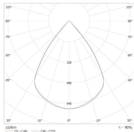
KANLUX S.A. (kat 33980) AL-ML-NW-RST-W-NT / Krzywa rozsyłu światła (biegunowo)
