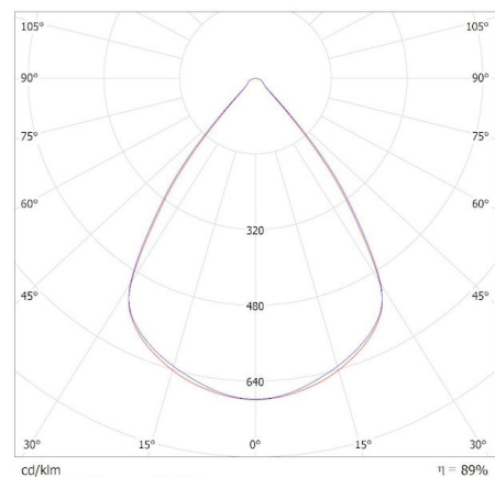
KANLUX S.A. (kat 33982) AL-ML-WW-RST-W-NT / Krzywa rozsyłu światła (biegunowo)
