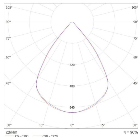
KANLUX S.A. (kat 33983) AL-MH-WW-RST-W-NT / Krzywa rozsyłu światła (biegunowo)
