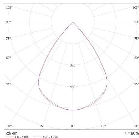
KANLUX S.A. (kat 33993) AL-MH-NW-RST-B-NT / Krzywa rozsyłu światła (biegunowo)
