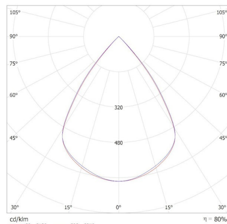
KANLUX S.A. (kat 33995) AL-MH-WW-RST-B-NT / Krzywa rozsyłu światła (biegunowo)
