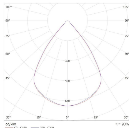
KANLUX S.A. (kat 34049) AL-MM-WW-RST-W-NT / Krzywa rozsyłu światła (biegunowo)
