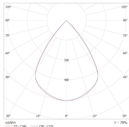
KANLUX S.A. (kat 34055) AL-MM-WW-RST-B-NT / Krzywa rozsyłu światła (biegunowo)
