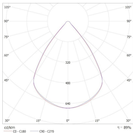
KANLUX S.A. (kat 34090) AL-LL-WW-RST-W-NT / Krzywa rozsyłu światła (biegunowo)
