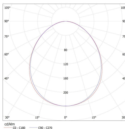
KANLUX S.A. (kat 27413) ALIN 4LED 1X120-W + GLASSv3 / LDC (Polar)
