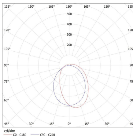
KANLUX S.A. (kat 28662) FT1500 55W-840-ASY / LDC (Polar)
