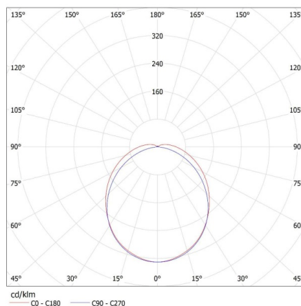
KANLUX S.A. (kat 28871) FTHT1500 43W-840-RYF / LDC (Polar)
