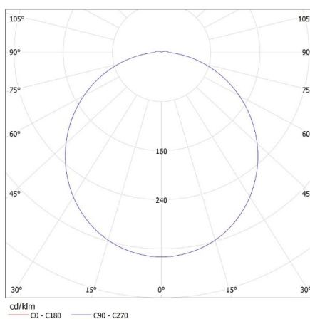
KANLUX S.A. (kat 33341) BENO 24W NW-O-GR / LDC (Polar)
