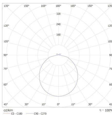
KANLUX S.A. (kat 35257) IQ-LED GU10 4,9W-NW / Krzywa rozsyłu światła (biegunowo)
