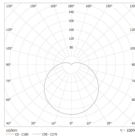
KANLUX S.A. (kat 36689) IQ-LED G45E14 3,4W-NW / Krzywa rozsytu światła (biegunowo)
