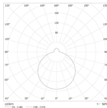
KANLUX S.A. (kat 37330) ARVOS LED 37W CCT B / Krzywa rozsyłu światła (biegunowo)
