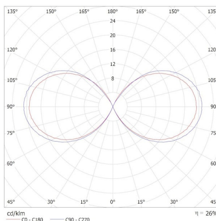
KANLUX S.A. (kat 38768) DASTEN EL16 S SO B / Krzywa rozsyłu światła (biegunowo)
