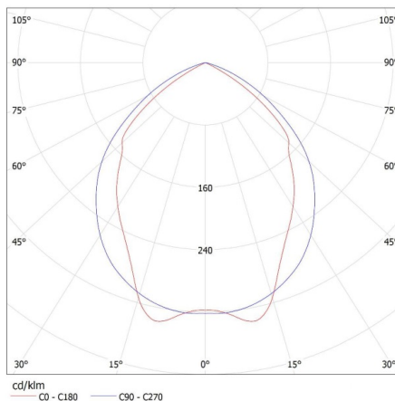
KANLUX S.A. (kat 22671) NOTUS 4LED 418 NT + T8 Miledo / Krzywa rozsyłu światła (biegunowo)
