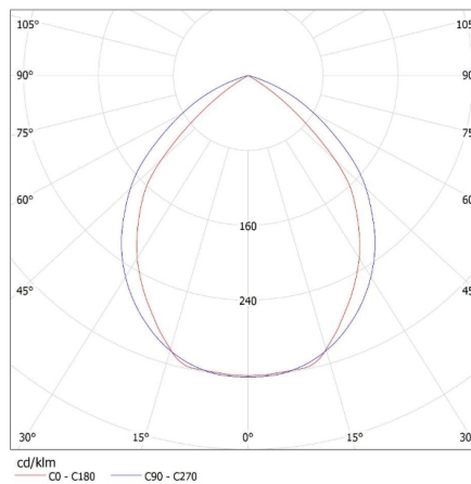
KANLUX S.A. (kat 22672) NOTUS 4LED 236 NT + GLASSv3 / LDC (Polar)
