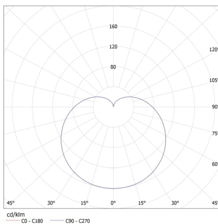
KANLUX S.A. (kat 23422) BILO 6,5W T SMD E14-WW / Krzywa rozsyłu światła (biegunowo)
