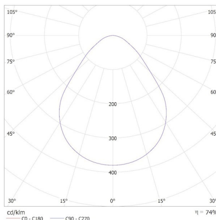
KANLUX S.A. (kat 26381) TIBERI CCT 15-21W-W 4000K / Krzywa rozsytu światła (biegunowo)
