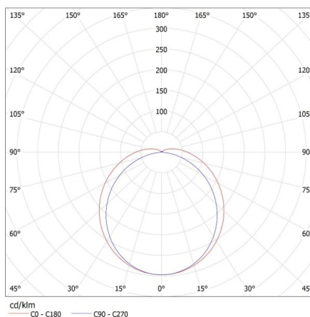
KANLUX S.A. (kat 28858) FT1500 43W-840-OPL / LDC (Polar)
