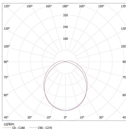
KANLUX S.A. (kat 28867) FTHL1500 73W-840-RYF / LDC (Polar)
