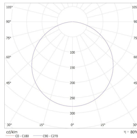
MLEDO (kat 31173) BAREV BL LEDN2 40W-NW / Krzywa rozsyłu światła (biegunowo)
