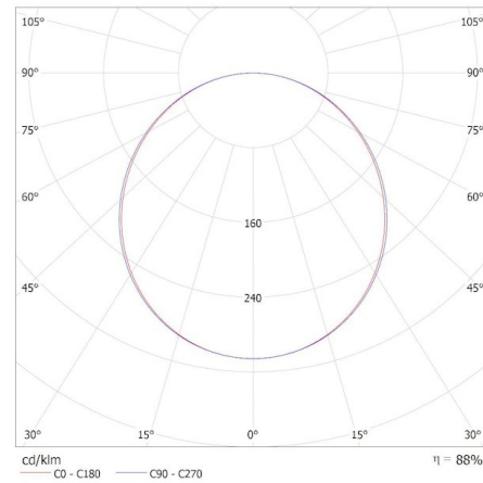
MILED o (kat 31174) BAREV BL 40W 12030 NW / Krzywa rozsyłu światła (biegunowo)
