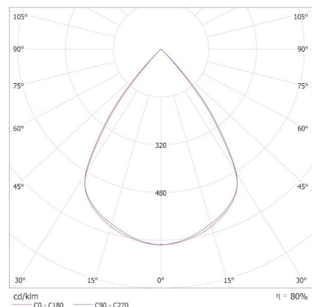
KANLUX S.A. (kat 34054) AL-MM-NW-RST-B-NT / Krzywa rozsyłu światła (biegunowo)
