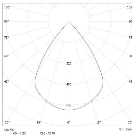
KANLUX S.A. (kat 36150) OS-L8D-WN-RST-B-N1 / Krzywa rozsyłu światła (biegunowo)
