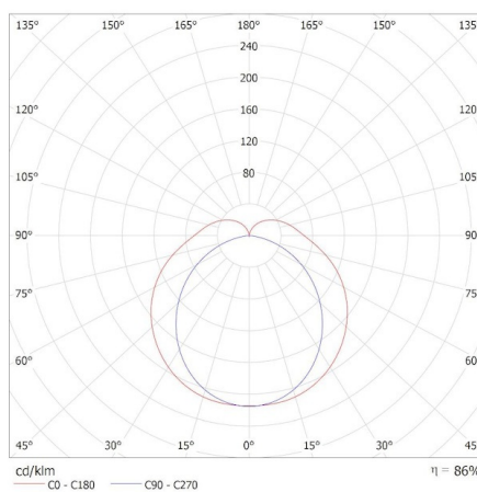
KANLUX S.A. (kat 36661) AKVO IP44 15W-NW-C / Krzywa rozsyłu światła (biegunowo)
