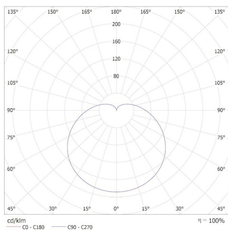
KANLUX S.A. (kat 36675) IQ-LED A60 5,9W-CW / Krzywa rozsytu światła (biegunowo)
