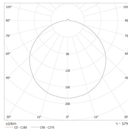
KANLUX S.A. (kat 37317) NIFU LED17,8W NW_BR / Krzywa rozsyłu światła (biegunowo)
