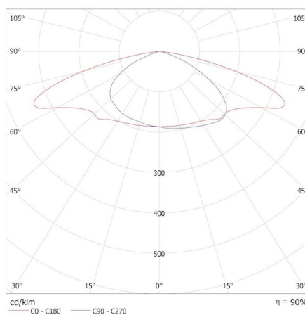
KANLUX S.A. (kat 39286) PRO-S M 100W NW / Krzywa rozsyłu światła (biegunowo)
