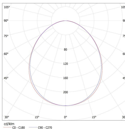
KANLUX S.A. (kat 27421) ALIN 4LED 1X120-SR-NT + GLASSv3 / LDC (Polar)
