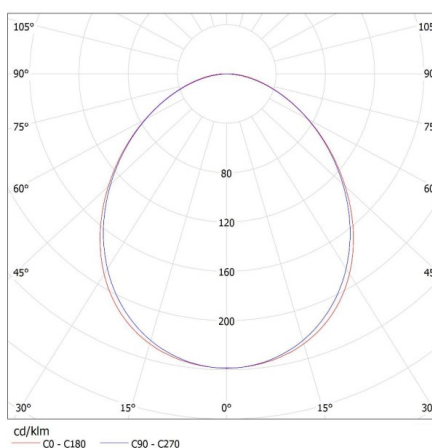
KANLUX S.A. (kat 27426) ALIN 4LED 1X150-B-NT + GLASSv3 / LDC (Polar)
