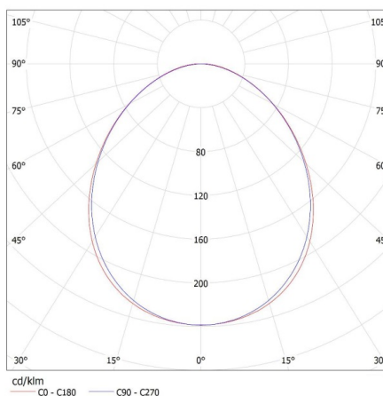
KANLUX S.A. (kat 27427) ALIN 4LED 1X150-SR-NT + GLASSv3 / LDC (Polar)
