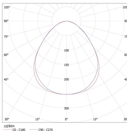
KANLUX S.A. (kat 28444) AL 4LED 60-MPR-B + GLASSv3 / LDC (Polar)
