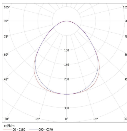
KANLUX S.A. (kat 28454) AL 4LED 150-MPR-SR-NT + GLASSv3 / LDC (Polar)
