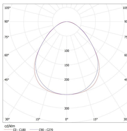
KANLUX S.A. (kat 28456) AL 4LED 150-MPR-B + GLASSv3 / LDC (Polar)
