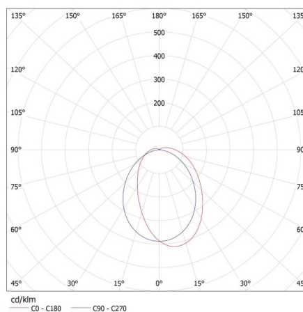
KANLUX S.A. (kat 28634) FT1200 37W-840-ASY / LDC (Polar)
