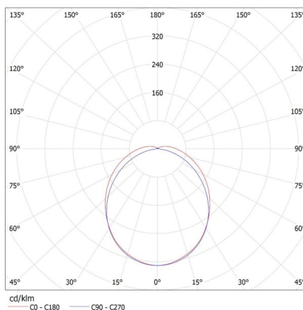
KANLUX S.A. (kat 28871) FTHT1500 43W-840-RYF / LDC (Polar)
