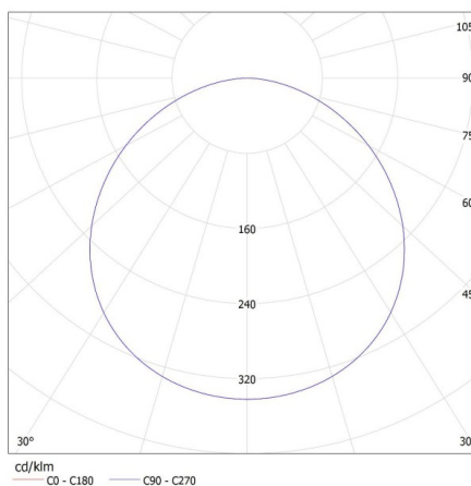
KANLUX S.A. (kat 28951) KANTI V2LED 18W-NW-W / LDC (Polar)
