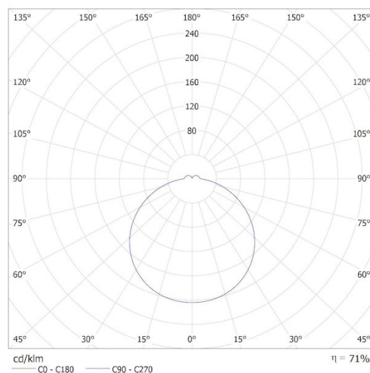
MILEDO (kat 31241) DUNO PRO 24W-NW-O / Krzywa rozsyłu światła (biegunowo)
