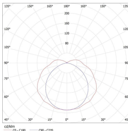
KANLUX S.A. (kat 22801) MAH PLUS-258/4LED/ i GLASSv2 / Krzywa rozsyłu światła (biegunowo)
