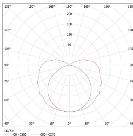
KANLUX S.A. (kat 22802) MAH PLUS-136/4LED/PC + Miledo / LDC (Polar)
