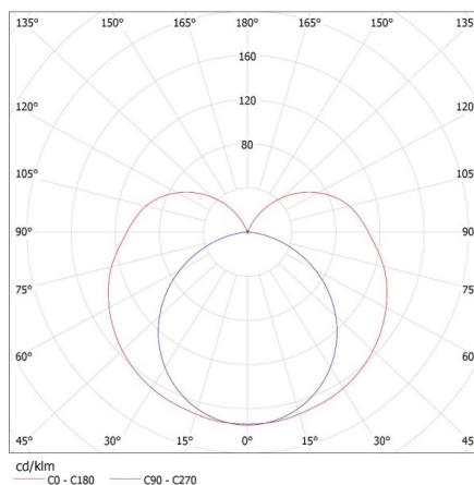
KANLUX S.A. (kat 26360) ALDO 4LED 1X60 + GLASSv2 / Krzywa rozsyłu światła (biegunowo)
