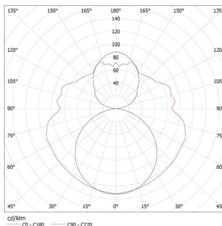
KANLUX S.A. (kat 26364) ALDO 4LED 2X120 + GLASSv2 / Krzywa rozsyłu światła (biegunowo)
